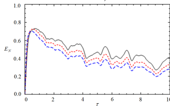
شکل ۳: نمودار منفیت بر حسب \tau برای نور چلانده به ازای \gamma/\lambda = 0.01 برای \bar{n} = 8 (خط توپر سیاه)، \bar{n} = 16 (نقطه چین قرمز)، و \bar{n} = 24 (خط چین آبی).
