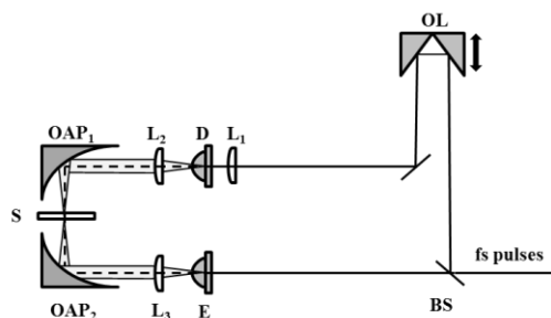
شکل ۱: چیدمان آزمایشگاهی طیف‌نگار عبوری ترارتر. در این چیدمان BS تقسیم‌کننده نوری، OL تأخیر انداز نوری، L_1 عدسی نوری، D و E به ترتیب آنتن فرستنده و گیرنده، L_2 و L_3 عدسی‌های TPX، OAP_1 و OAP_2 آینه‌های سهموی و S نشانگر نمونه است.
