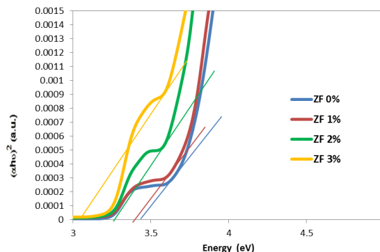
شکل (۴) - نمودار گاف انرژی لایه‌های اکسیدروی آلاییده با درصد‌های مختلف
