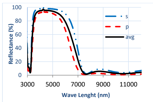
شکل ۲: طیف های بالا مربوط به اندازه گیری پوشش پرتوشکاف ساخته شده نهایی می باشد. این طیف های بازتاب نسبی، مربوط به قطبش s، قطبش p و متوسط قطبش s و p می باشد و در دستگاه FTIR و نسبت به طلا در زاویه ۴۵ درجه گرفته شده است.
