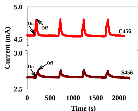
شکل ۶: پاسخ نوری دینامیکی نمونه های C456 و S456 به تابش نور قرمز با طول موج ۶۲۰ nm.
