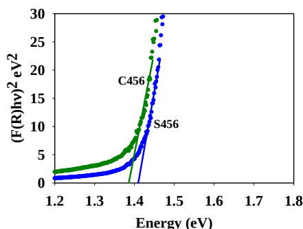
شکل ۴: تحلیل داده‌های اپتیکی در نمونه‌های تحت بررسی مبتنی بر معادله ۲.
