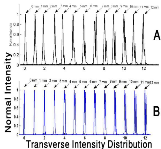
شکل ۹: مقایسه نتایج تئوری و تجربی برای توزیع شدت عرضی صفحه کانون برای تمام نمونه‌ها. نمودار حاصل از A: داده‌های تجربی و B: داده‌های شبیه سازی. تمام توزیع شدت‌ها به یک نرمال شدند اند.
