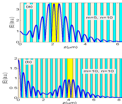
شکل ۵: توزیع میدان الکتریکی در \lambda_p = 1.326 \mu m : (a) m=5, n=10 و (b) m=10, n=10 را نشان می‌دهند.
