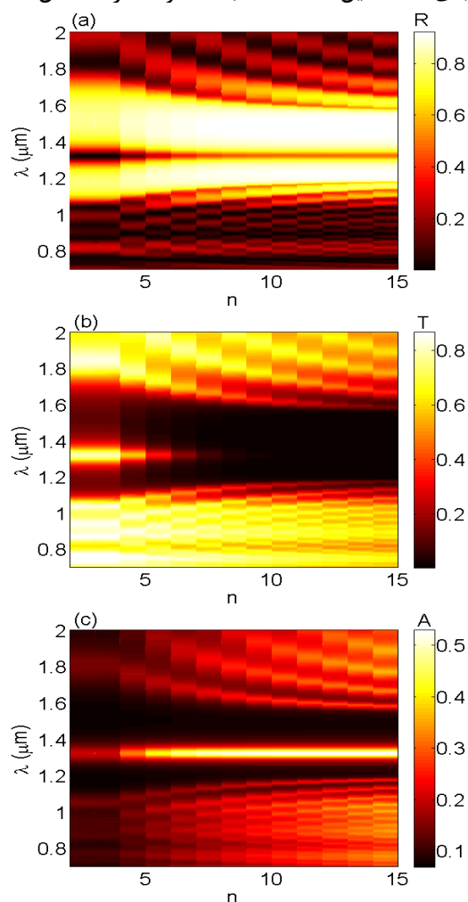
شکل ۲: طیف بازتابندگی (a)، تراگیسلندگی (b) و جذب (c) در صفحه‌ی \lambda - n برای m=3 . در اینجا \mu_c = 0.2 \text{ eV} و T = 20^\circ\text{C} می‌باشند.
