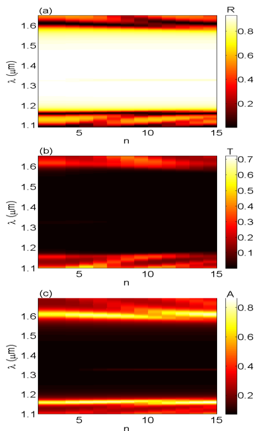
شکل ۴: طیف بازتابندگی (a)، تراگسیلندگی (b) و جذب (c) در صفحه‌ی n-\lambda برای m=10 . در اینجا \mu_c = 0.2 \text{ eV} و T = 20^{0C} می‌باشند.
