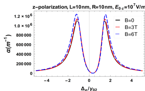
شکل ۲: ضریب جذب خطی در حضور و عدم حضور میدان مغناطیسی و قطبش در جهت Z
