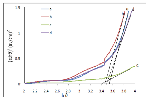
شکل ۳: تعیین گاف انرژی لایه های نازک \text{SnO}_2 بازپخت شده در دماهای (a) 650^\circ\text{C} ، (b) 550^\circ\text{C} ، (c) 450^\circ\text{C} بدون بازپخت (d) 550^\circ\text{C}
