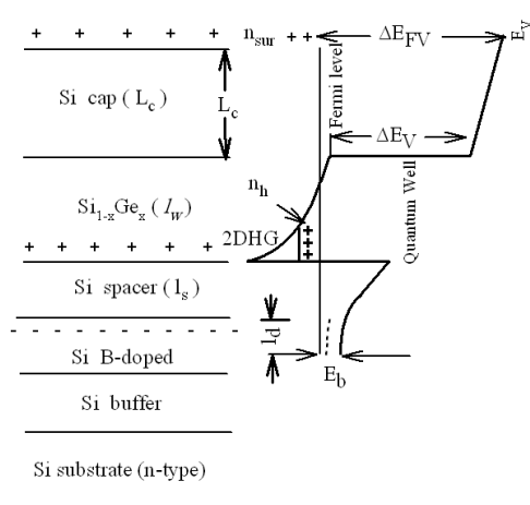
کل (۱) ترتیب رشد لایه‌ها و ساختار نوار ظرفیت در ساختار مورد مطالعه
