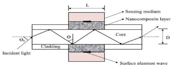
شکل ۱: شماتیک از سنسور فیبر نوری SPR
