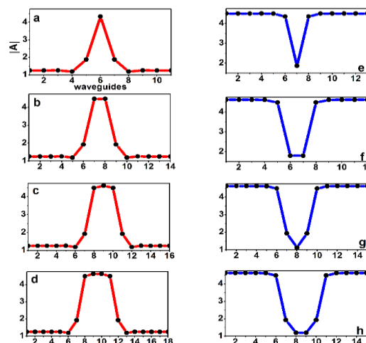
شکل ۳: پروفایل چند نمونه از سالیتون‌های کاواک گسسته‌ی روشن (سمت چپ) و تاریک (سمت راست) با P = 4 .
