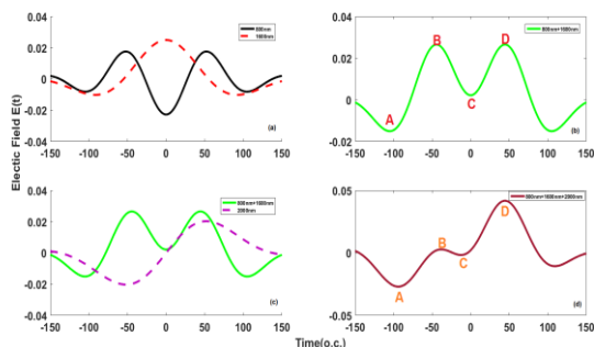
شکل ۱: (a) ترکیب دو میدان تک رنگ \lambda = 1600nm و \lambda = 800nm (b) میدان دو رنگ \lambda = 1600nm + 800nm (c) ترکیب میدان دو رنگ و تک رنگ \lambda = 2000nm (d) میدان سه رنگی \lambda = 800 + 1600 + 2000nm
