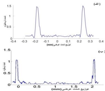
شکل ۷: نمودار تجربی توزیع شدت عرضی CFZP برای: الف) m=0/5 و n=0 ، ب) m=2/5 و n=0 .
