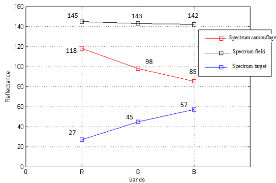
شکل ۴: طیف (بردار طیفی) استتار، طیف هدف و طیف زمینه را برای پیکسلی که در شکل ۴ (الف) و (ب) مشخص شده است.
