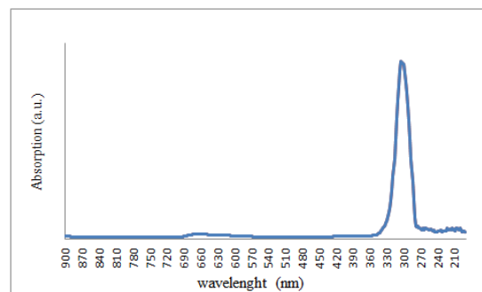
شکل ۳: طیف UV- visible بلوئومایسین
