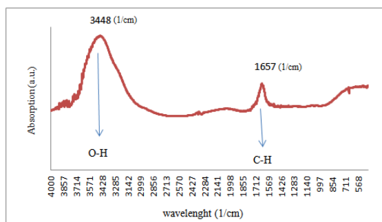
شکل ۷: طیف FTIR وینکریستین
