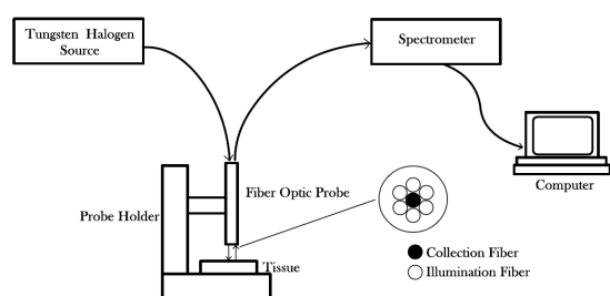
شکل ۱: طرح‌واره‌ای از چیدمان طیفسنجی بازتابی پخش.
