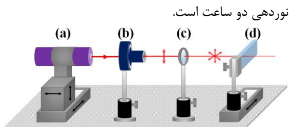
شکل ۱- طرحواره‌ای از چیدمان نوردهی نمونه Ag-AgCl، (a) لیزر و نگهدارنده آن، (b) قطبشگر گلان-تیلور، (c) دی‌پلاریزور و (d) نمونه.
