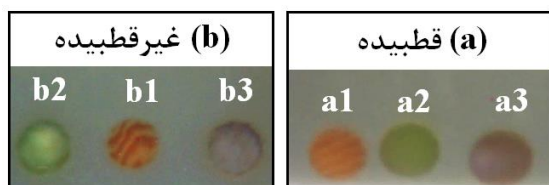
شکل ۲- لایه‌ی Ag-AgCl بعد از نوردهی با پرتوهای (a) قطبیده و (b) غیرقطبیده، لیزر هلیوم-نئون (a1, b1)، لیزر Nd:YAG (a2, b2) و لیزر دیودی بنفش (a3, b3).
