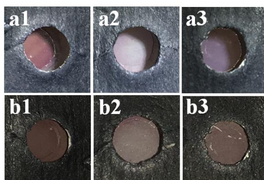
شکل ۶- لایه Ag-AgCl (a) قبل از تابش نور سفید و (b) بعد از تابش نور سفید. نقاط a1 و b1 با پرتوهای لیزر هلیوم-نئون، a2 و b2 با لیزر Nd:YAG و a3 و b3 با لیزر دیودی بنفش نوردهی شده است.
