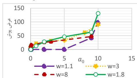
شکل ۵: بررسی تغییرات عرض پوش سالیونی بر حسب a_0
