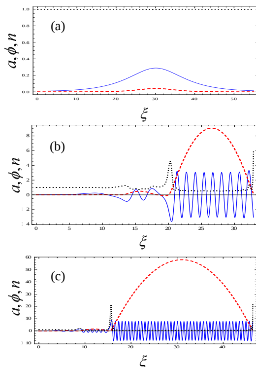
شکل ۶: پتانسیل برداری نرمالیزه میدان الکتریکی لیزر a (خط آبی رنگ)، پتانسیل اسکالر نرمالیزه الکترواستاتیک wake field \phi (خط قرمز رنگ) و چگالی الکترون n (نقطه چین مشکی رنگ) بر حسب \xi برای حالت (a) \varepsilon=0/3, a_0=9 (b) \varepsilon=0/9, a_0=0/1 (c) \varepsilon=0/2867, a_0=10
