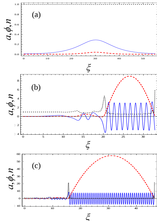
شکل ۲: پتانسیل برداری نرمالیزه میدان الکتریکی لیزر a (خط آبی رنگ)، پتانسیل اسکالر نرمالیزه الکترواستاتیک wake field \phi (خط قرمز رنگ) و چگالی الکترون n (نقطه چین مشکی رنگ) بر حسب \xi برای حالت (a) \varepsilon=0/3, \omega=5 (b) \varepsilon=0/9, \omega=1/1 (c) \varepsilon=0/199, \omega=9
