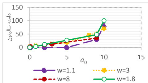
شکل ۳: بررسی تغییرات دامنه سالیون بر حسب a_0
