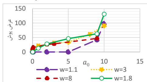
شکل ۸: بررسی تغییرات عرض پوش سالیتونی بر حسب a_0
