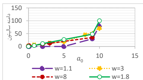
شکل ۷: بررسی تغییرات دامنه سالیتون بر حسب a_0
