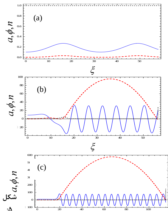
شکل ۵: پتانسیل برداری نرمالیزه میدان الکتریکی لیزر a (خط آبی رنگ)، پتانسیل اسکالر نرمالیزه الکترواستاتیک wake field \phi (خط قرمز رنگ) و چگالی الکترون n (نقطه چین مشکی رنگ) بر حسب \xi برای حالت (a) \varepsilon=0/3, a_0=9 (b) \varepsilon=0/9, a_0=0/1 (c) \varepsilon=0/2867, a_0=10
