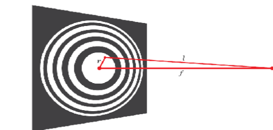
شک ۱: نقطه‌ی منبع در ناحیه‌ی اول و فاصله‌ی کانونی f و طول راه نوری l
