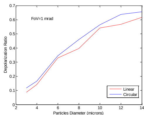
شکل ۳: تغییرات ضریب واقطبش خطی و دایروی برحسب قطر ذرات برای یک لایه ابر به ضخامت ۱۰۰ متر و چگالی عددی (cm^{-3}) و به ازاء میدان دید ۱ میلی رادیان
