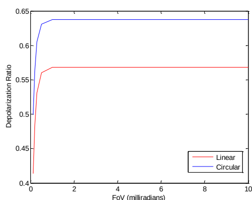
شکل ۴: تغییرات ضریب واقطبش خطی و دایروی برحسب زاویه میدان دید گیرنده لیدار برای یک لایه ابر به ضخامت ۱۰۰ متر و چگالی عددی (cm^{-3}) و متشکل از قطرات آب به قطر ۱۲ میکرون
