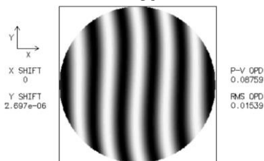
شکل ۸: الگوی تداخلی در نتیجه‌ی اعمال خطا به میزان
