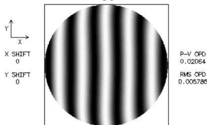
شکل ۱۲: الگوی تداخلی در نتیجه‌ی اعمال خطا به میزان 0.05mm در شعاع سطح غیرکروی عدسی جبران کننده
