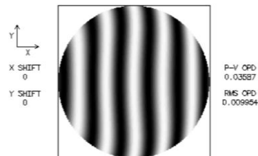
شکل ۶: الگوی تداخلی در صورت خروج از تفرانس ضخامت مرکزی
