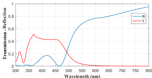
شکل ۴: ضرایب بازتاب (نمودار آبی) و عبور (نمودار قرمز) ساختار فراماده هایپرپولیک
