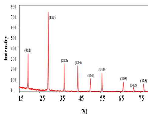
شکل ۱- الگوی پراش اشعه ایکس \text{LaAlO}_3 تهیه شده به روش تعامل حالت جامد و شوک حرارتی (شدت پیک بر حسب 2\theta زاویه پراش). الگوی پراش ثبت و ضبط شده کاملاً منطبق با پوشه ذریع در کتابخانه (JCPDS 31-0022) می باشد.
