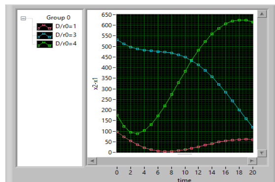
شکل (۶) نمودار تغییر مکان ورتکس با زمان مربوط به پرتو ایری دارای ورتکس برای سه حالت با D/r_0 مختلف است.
