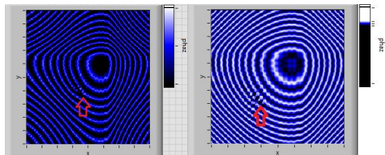
شکل (۲) نمودار فاز پرتو ابری معمولی دارای ورتکس و نمودار ابری تحت تبدیل فوریه کسری دارای ورتکس به ازای p=0.5 و z=1000mm است.
