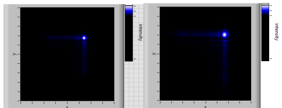
شکل (۳) نمودار شدت پرتو ابری معمولی دارای ورتکس و نمودار ابری تحت تبدیل فوریه کسری دارای ورتکس به ازای p=0.5 و z=1000mm است.
