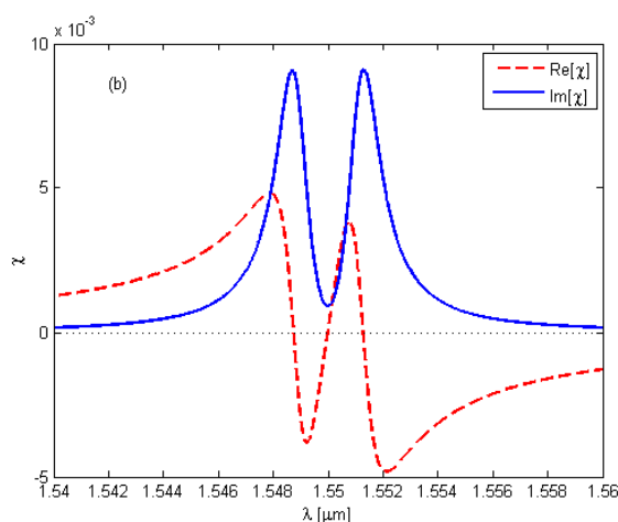
شکل ۲. نمودار جذب و پاشندگی به ازای پارامترهای
