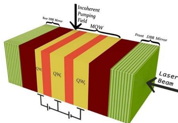
شکل ۱ سیستم چاه کوانتومی سه گانه از جنس InGaAs/InP
