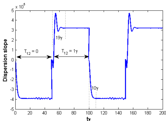
شکل ۳ نمودار کلیدزنی سرعت گروه بر اساس تونل زنی به ازای
