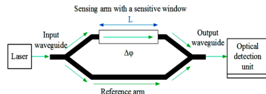
شکل ۳: تداخل سنج ماخ ذندر و مسیر عبور نور در بازوها [۸].
