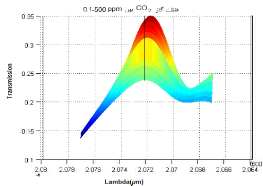
شکل ۶: طیف خروجی و شیف فرکانسی به ازای تغییرات در غلظت CO 2 .
