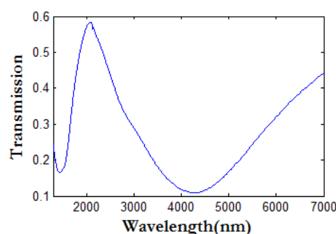
شکل ۲: نمودار عبور برای رزوناتور نانودیسک‌های تک لایه GZO
