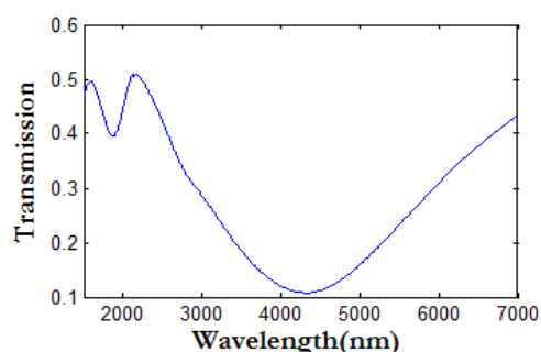
شکل ۳: نمودار عبور برای رزوناتور نانودیسک‌های دو لایه GZO/ZnO
