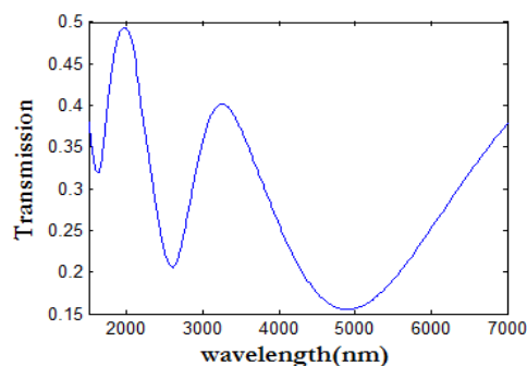
شکل ۴: نمودار عبور برای رزوناتور نانودیسک‌های سه لایه GZO/ZnO
