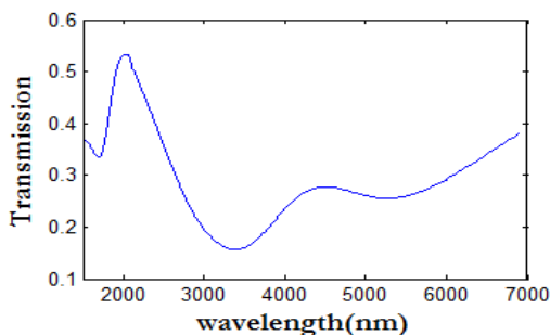
شکل ۵: نمودار عبور برای رزوناتور نانودیسک‌های چهار لایه GZO/ZnO
