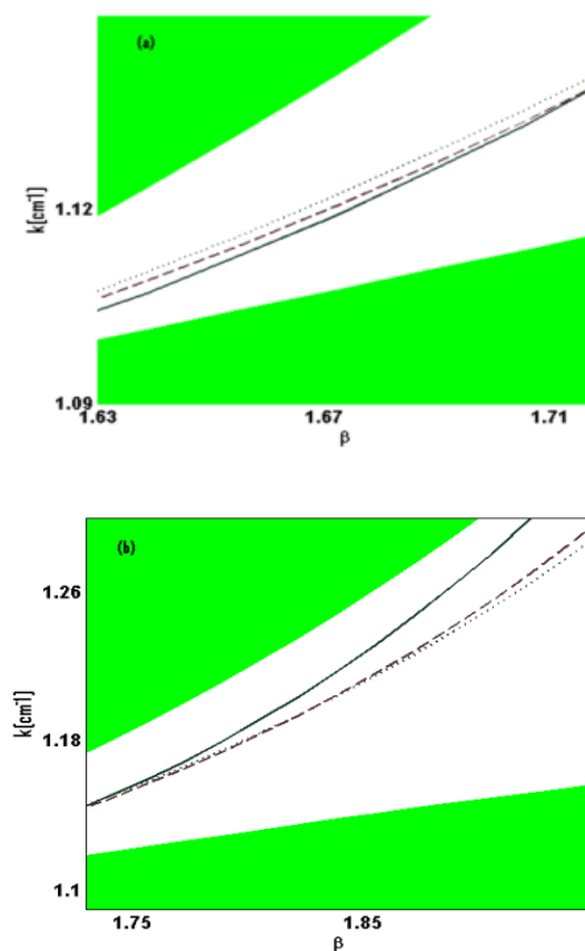
شکل ۳: منحنی پاشندگی امواج سطحی TM در حضور تیغه خود-واکانونی کننده روی صفحه (k, \beta) در اولین نوار ممنوعه بلور فوتونی حاوی فراماده به ازای \gamma_0 = -0.5 : الف: 1.63 < \beta < 1.73 و ب: 1.73 < \beta < 1.94 . منحنی های نقطه چین، خط چین و توپر پاشندگی امواج سطحی را به ترتیب به ازای d_s = 3d_1, 2d_1, 1.5d_1 نشان می دهد.
