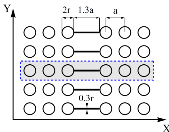
شکل ۱: طرح واره موجبر بلور فوتونی برای توقف کامل نور. مستطیل خط چین سلول واحد شبکه را نمایش می دهد.
