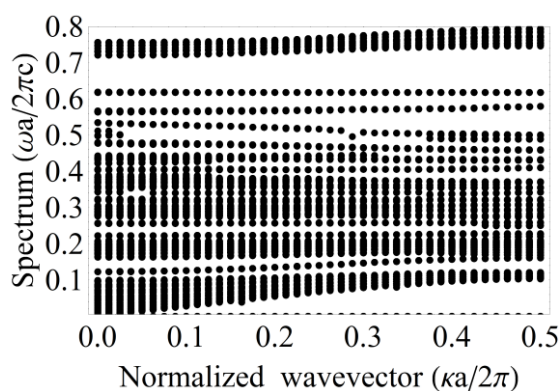
شکل ۲: ساختار نواری تصویر شده موجبر بلور فوتونی با ثابت شبکه ۴۵ میکرومتر و نسبت پر شدگی ۰/۳. در بسامد نرمالیزه ۰/۶۱۷ نوار هدایتی با شیب صفر در سراسر مولفه بردار موج در راستای انتشار تولید می شود.
