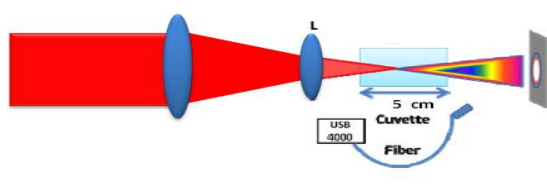
شکل ۱: نمایش طرح وار چیدمان آزمایشگاهی برای تولید ابرپیوستار
