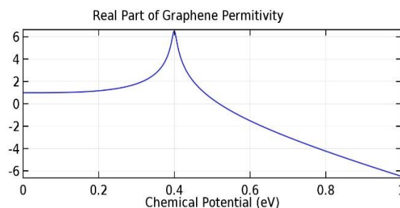
نمودار (۱) قسمت حقیقی گذردهی گرافن بر حسب پتانسیل شیمیایی، برای انرژی فوتون با طول موج 1550 nm
