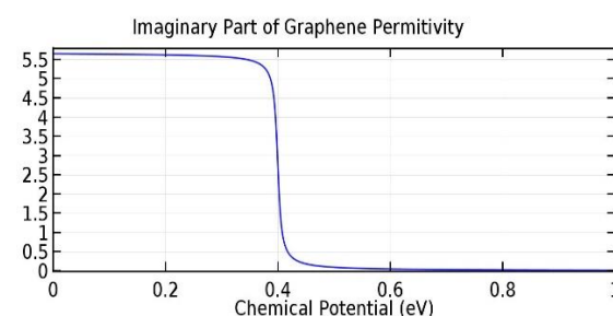
نمودار (۲) قسمت موهومی گذردهی گرافن بر حسب پتانسیل شیمیایی، برای انرژی فوتون با طول موج 1550 nm
