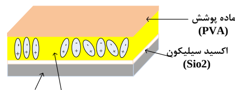
شکل ۳: شکل لایه‌های فیلم نازک پلیمر برای ساخت موجبر مایخزنر. کروموفر آزو زیر پایه سیلیکون
